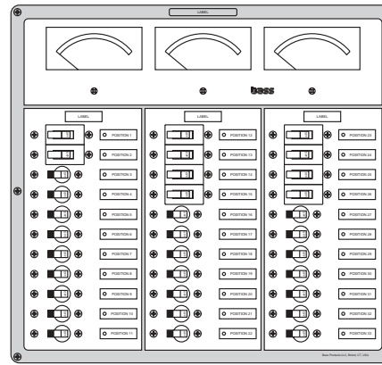
90-9130 14.5"W x 13.5"H x 3.5"D
