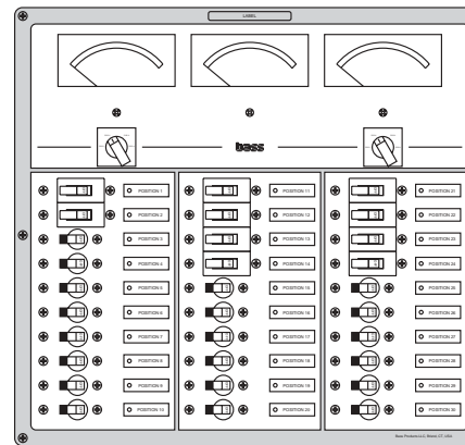
90-9170 14.5"W x 13.5"H x 3.5"D
