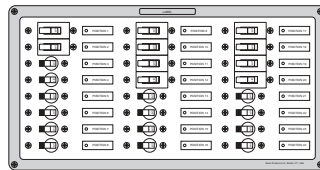
90-9134 14.5"W x 7.5"H x 3.5"D
