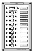
90-9115 5.5"W x 9"H x 3.5"D
