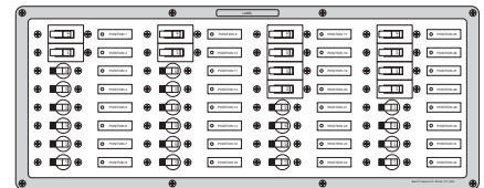
90-9144 19"W x 7.5"H x 3.5"D
