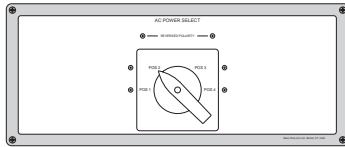
90-9330 14.5"W x 6"H x 3.5"D
