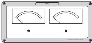
90-9502 10"W x 4.5"H x 3.5"D
