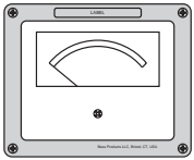
90-9501 5.5"W x 4.5"H x 3.5"D
